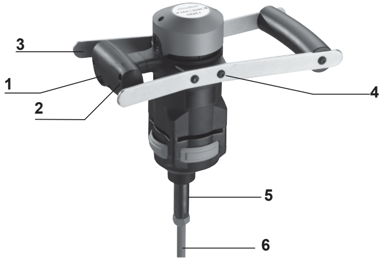
Das Rührwerk immer mit zwei Händen halten
